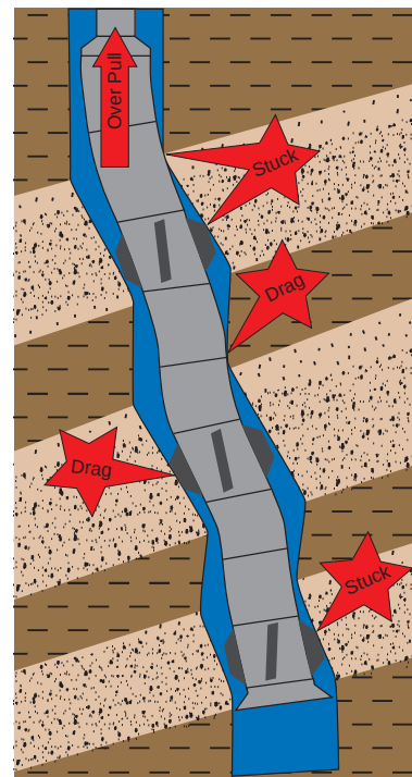
Doglegs
